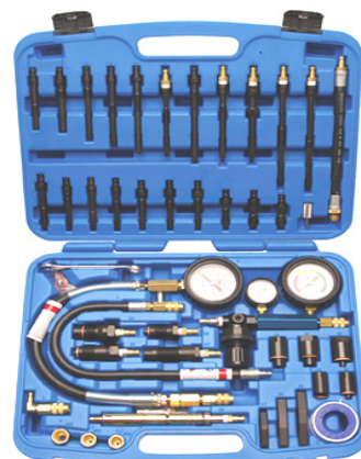
BGS8401 MASTER SET Compressiemeter en drukverlies tester benzine & diesel Compressiomètre et testeur de fuites de cylindres diesel et essence 493 €
