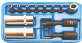
BGS2275 Demontageset voor airco. Set de démontage airco 2,2 - 3,2mm / 12 & 15mm 8 pans-kant / TS10-->40
