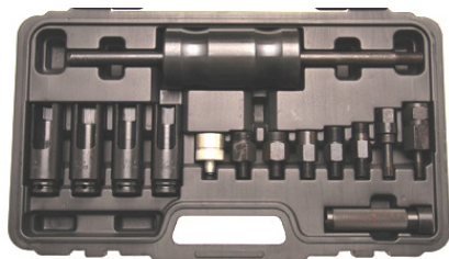
BGS67307 Verstuiwerstrekker extracteur d'injecteurs Adapter (Binnen-Intérieur): M14xM14-M17xM14-M25xM14 -M27x M14 Adapter (Buiten-extérieur):M27&M20xM14 Doppen-douilles 25 - 27 - 29 - 30 mm Semi-pro
