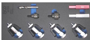
BGS9088 Set om de parking sensors in bumpers te monteren. Set de montage de capteurs de parking dans les pare-chocs Ø 18.2 & 26.0 mm
