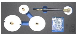
BGS9152 Adapters voor pour BGS8315 Bouchons Ø 90 Mitsubishi, Nissan, Subaru, Suzuki, Volvo S40, V40 - Ø 55 Chrysler, Ford Explorer, Hyundai, Mazda 6, Subaru - E20 Ford C-Max, Fiesta, Focus, Galaxy, S-Max
