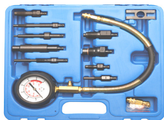
BGS8005 Compressiemeter benzine Compressiomètre essence 14 & 18mm 29 € BGS8236 12 & 14mm 29 € 0-21 bar
