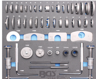
BGS1102 50 ST. / PCS. Terugstelset remzadelzuigers links-rechts 50-dlg. Set d'outils repousse piston de freins gauche-droite 50pcs
