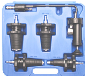
BGS8096 Koelsysteem tester Testeur du circuit de refroidissement Ø 17,0-60mm 0-2,4 bar
