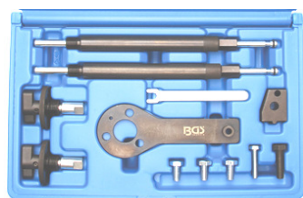
FIAT1 Kit de calage Afstelset Fiat 2.3D, 2.3 JTD / 3.0JTD - 3.0HDI
