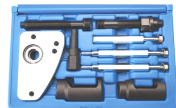
BGS8349 HDI Injectoren Bosch & Siemens Extracteur sans démonter la culasse / Trekkerset zonder montage cilinderkop PSA 2.0HDI DW10,DW12 Toyota,Mazda,Hyundai
