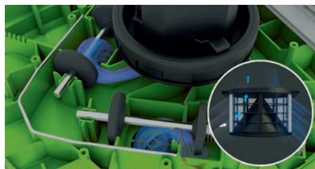
Filterreiniging door het omkeren van de luchtstroom Nettoyage du filtre par rétro-lavage du flux d'air
